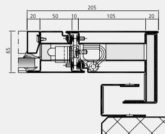
Schiebetür EI30 mit Fluchtweg-Funktion
