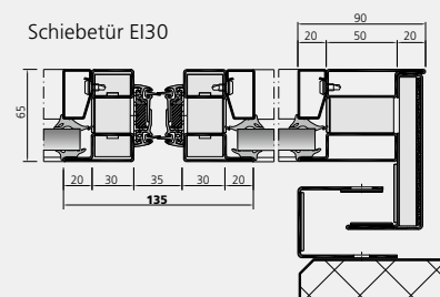
Schiebetür EI30 mit Fluchtweg-Funktion
