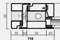
Verblechte Rohrrahmentür EI30/EI60
